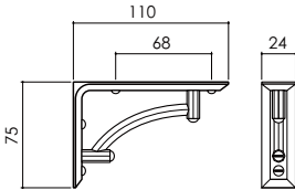
一般款（小） 代碼 TU-SN
