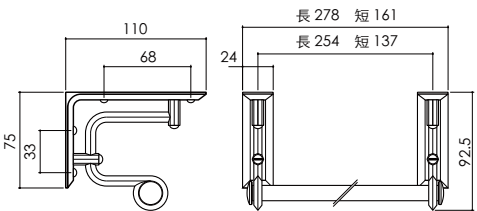
紙巾架款（短） 代碼 TU-SPS
