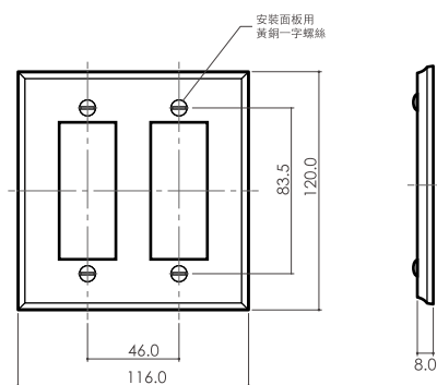
1112 二連四孔、六孔 代碼 CP-11-D
