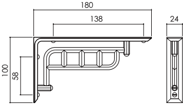
開孔款（中） 代碼 TU-MA
