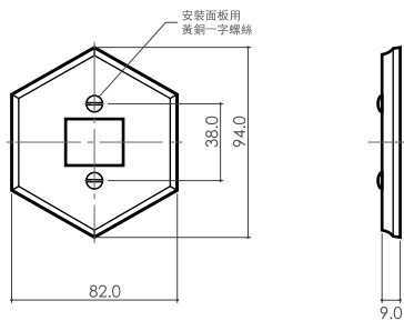
六角 一連一孔 代碼 CP-R-A
