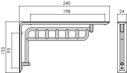
開孔款（大） 代碼 TU-LA
