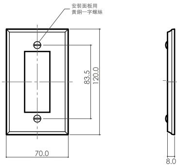
0712 一連二孔、三孔 代碼 CP-07-C
