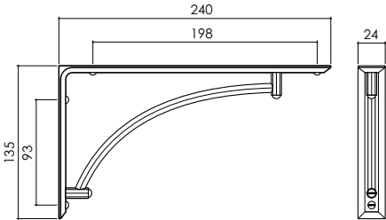
一般款（大） 代碼 TU-LN
