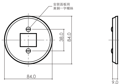
圓 一連一孔 代碼 CP-M-A
