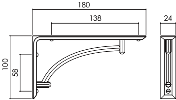
一般款（中） 代碼 TU-MN
