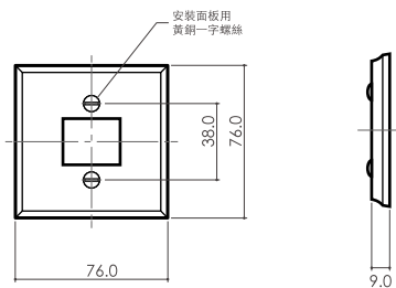
四角 一連一孔 代碼 CP-S-A
