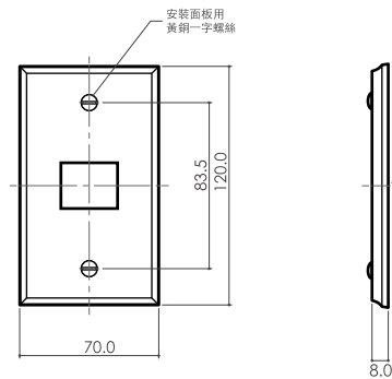
0712 一連一孔 代碼 CP-07-B
