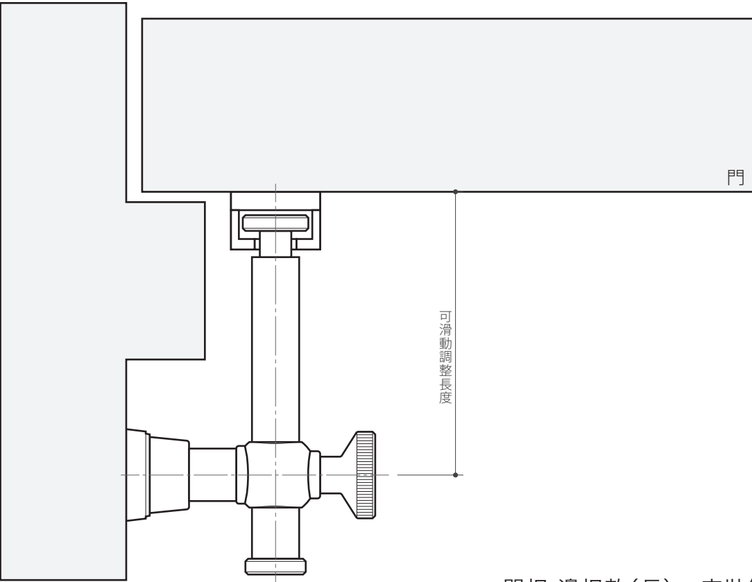
門扣 邊扣款(長) 安裝範例
