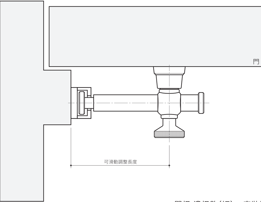
門扣 邊扣款(短) 安裝範例
